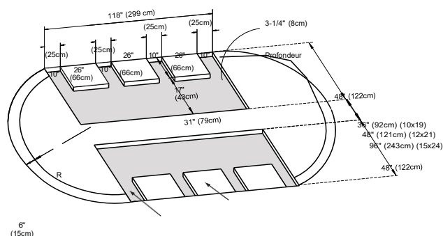
Surface du sol Tranchées pour dalles de ciment
