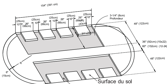
Surface du sol Tranchées pour dalles de ciment
